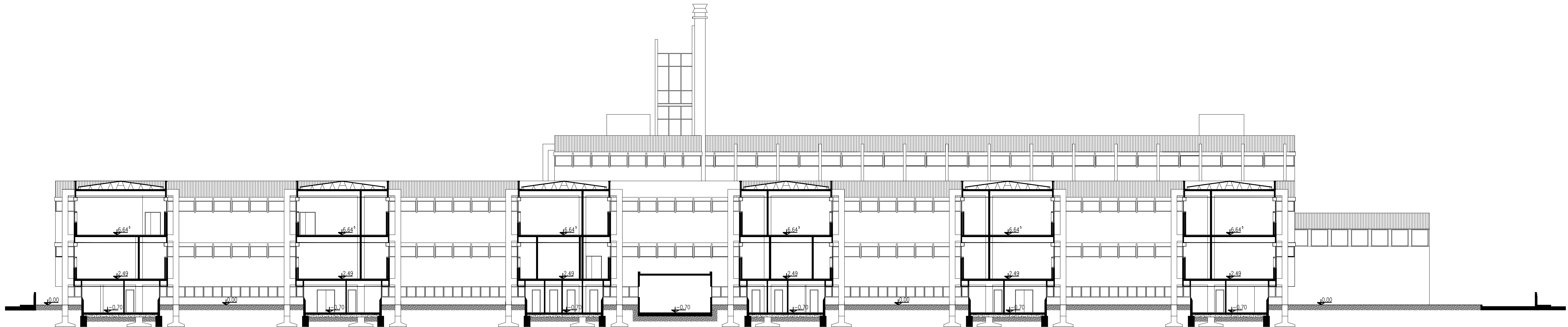
SEZIONE C-C
